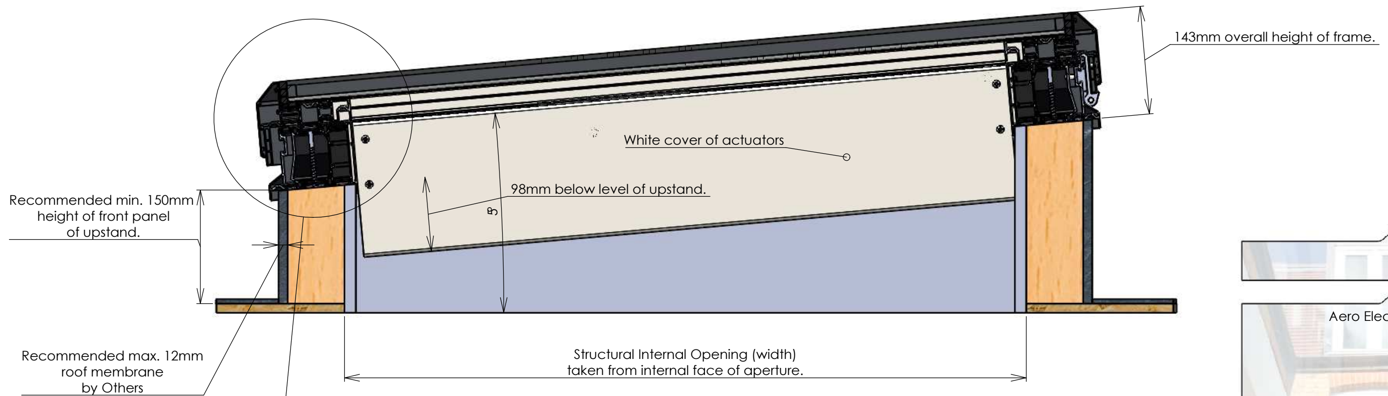
SECTION A-A
